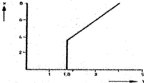
Figura 13 - Area sgombra intorno all'attrezzatura gonfiabile
